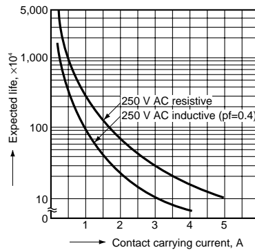
AC load (2C)
