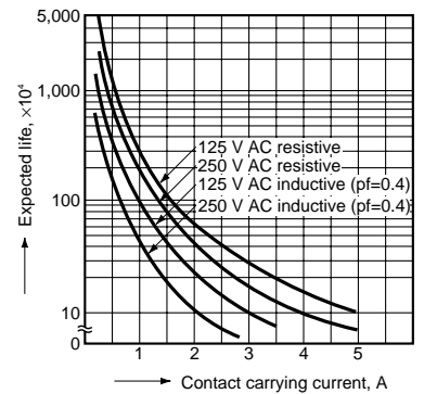
AC load (4C)
